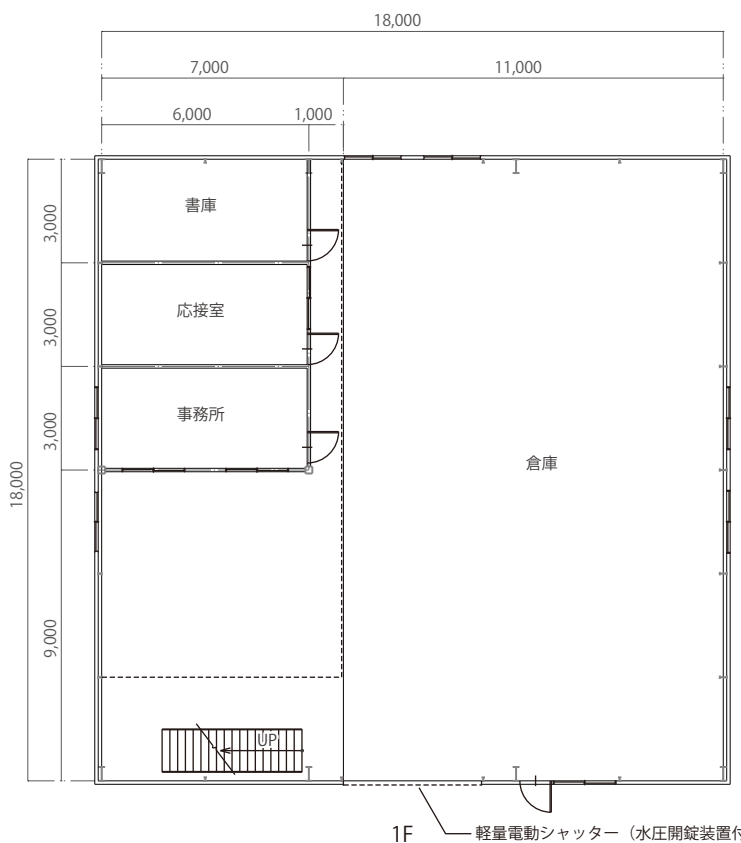
平面図
